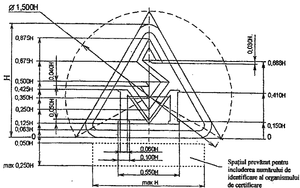
Figura 2. Dimensiunile mărcii naționale de conformitate SM
